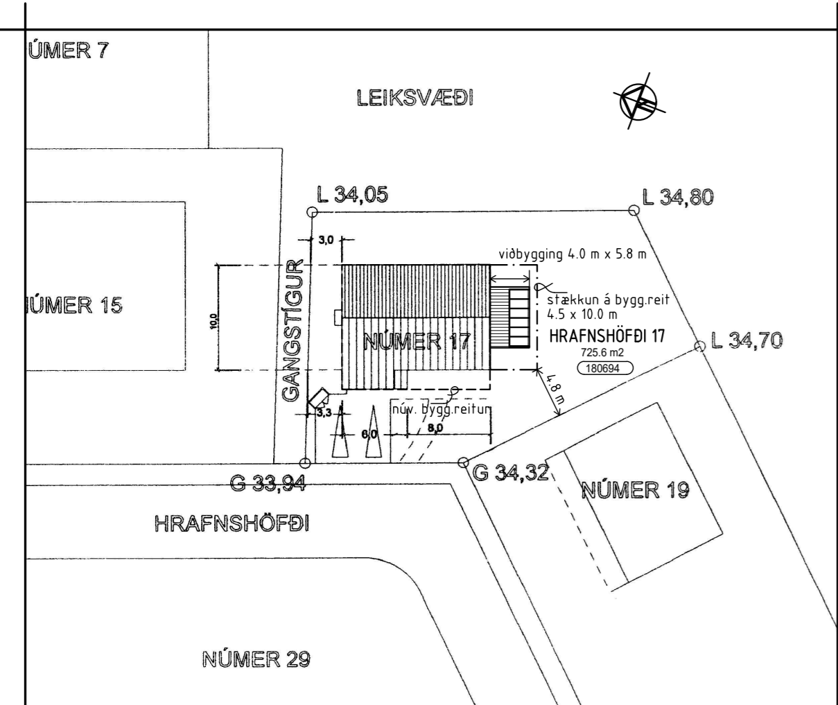
SKÝRINGARMYND mkv 1:500
